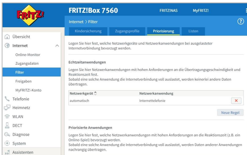
Abbildung 3 - Konfiguration der QoS-Regel
